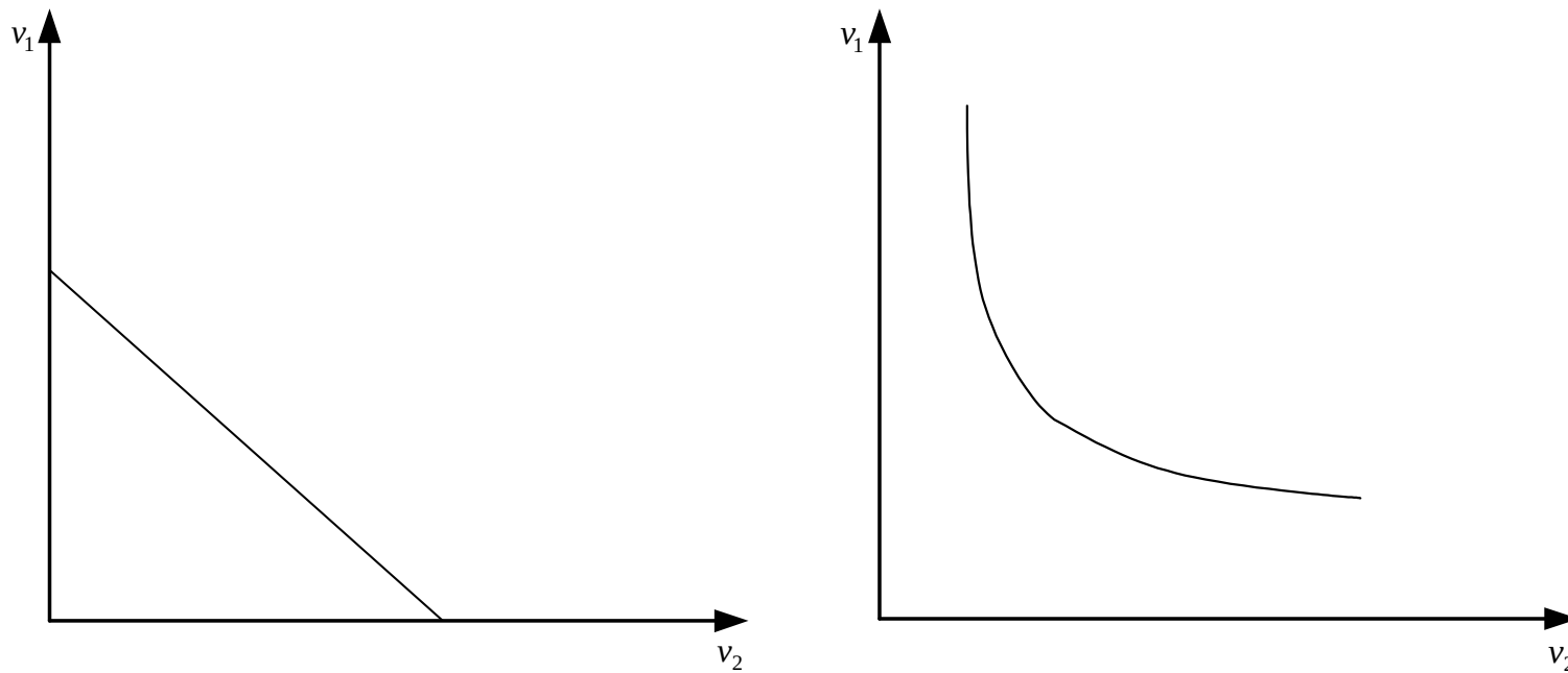
Abbildung 13.12-2: Dualität von Produktionsfunktion und Kostenfunktion
