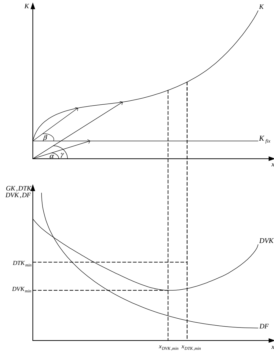
Abbildung 13.14-9: Typische Kostenkurve und zugehörige DTK-, DVK-, DF- und GK-Kurve
