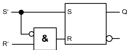
Abb. A.8: Beschaltung eines RS-Flipflops für vorrangigen S-Eingang
