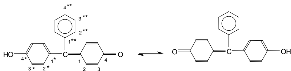
benzaurin
