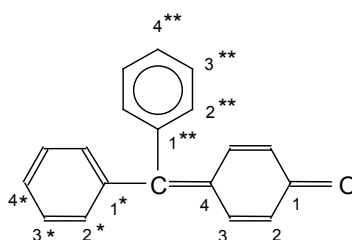
fuchsone
