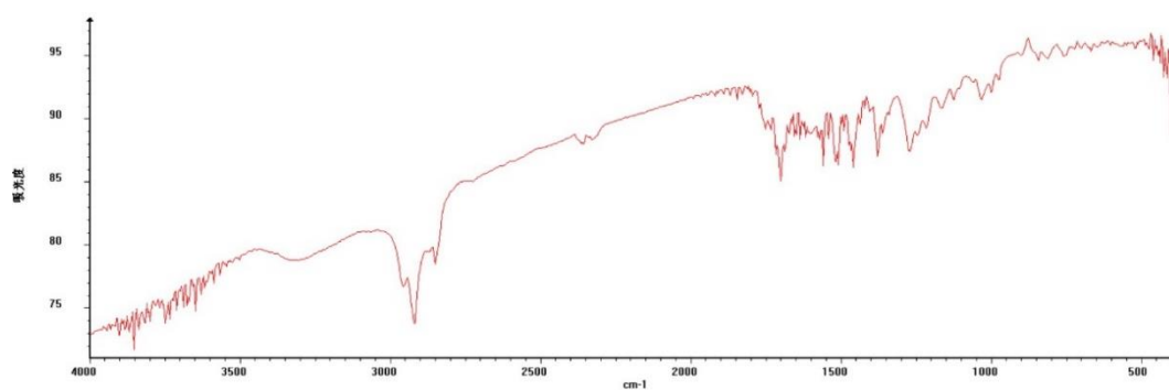
Fig. S3. IR (KBr) spectrum of oleraisoindole B in methanol- d_4
