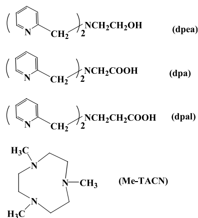
Scheme I.
