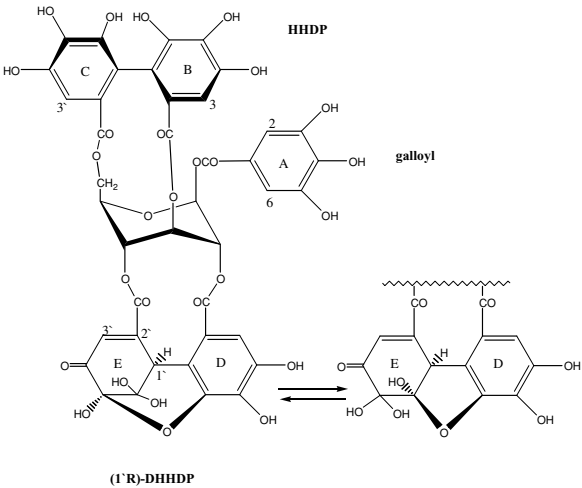
Fig. 1. Compound 2: Geraniin.
