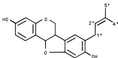
4: Sophorapterocarpin A (= 'Homoedudiol')
