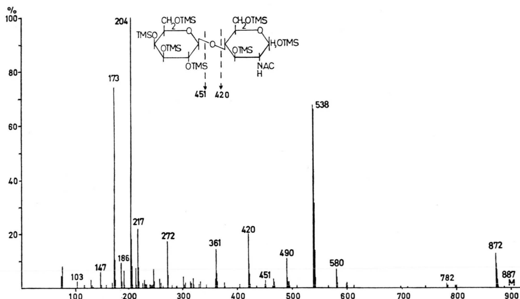
Abb. 6. 20 eV Massenspektrum der Pertrimethylsilyl-O- \beta -D-galaktopyranosyl-(1 \rightarrow 4)-D-N-acetylglucosamin, TMS-lactosamin.
