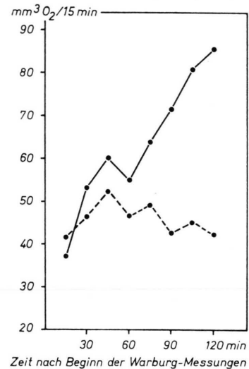
Abb. 2. Überleben der Bakterien nach Behandlung mit 8-MP (20 µg/ml) und UV (15 min aus 25 cm). Gemessen mm³ gebildeten O₂ pro 15 min in der Warburg-Apparatur. — Kontrolle ohne 8-MP und UV; --- Behandlung mit 8-MP und UV.
