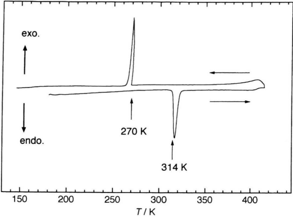
Fig. 1. DTA curve of \text{Li}_3\text{InBr}_6 .
