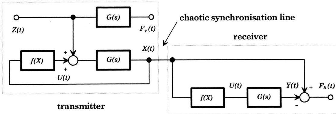
Fig. 3. The synchronisation principle.
