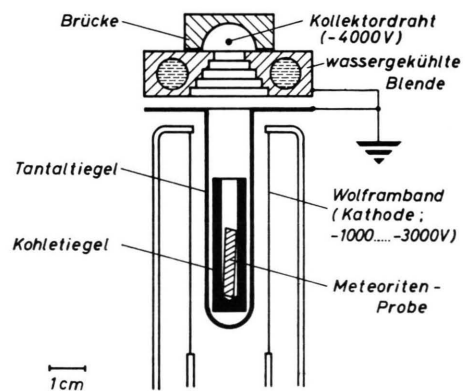
Abb. 3. Schema der Apparatur für die Extraktion von Kalium aus Eisenmeteoriten.
