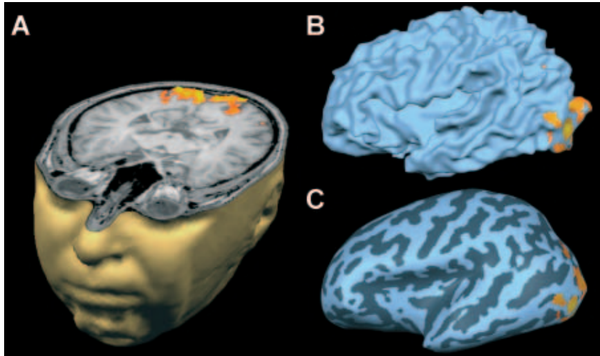
Abb. 6: Erweiterte Darstellungen der (A) koregistrierten funktionellen und anatomischen Daten (hier: der Intraparietalkortex) durch eine (B) Segmentierung und (C) anschließende Entfaltung des Gehirns, die nur noch der Oberfläche der grauen Hirnsubstanz entspricht (hellblau: Hirnwindungen, dunkelblau: Hirnfurchen).
