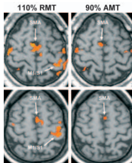
Abb. 7: Die Kombination der fMRT mit der transkraniellen Magnetstimulation (TMS) über dem primären motorischen Handareal führt bei überschwelliger Stimulation (links: 110% RMT) zu Aktivierungen der primären motorischen und sensorischen Areale (M1/S1) sowie des supplementären motorischen Areals (SMA). Im Gegensatz dazu aktiviert eine unterschwellige Stimulation (rechts: 90% AMT) nicht M1/S1, sondern nur das axonal verbundene SMA. Verändert aus Bestmann et al. (2003).
