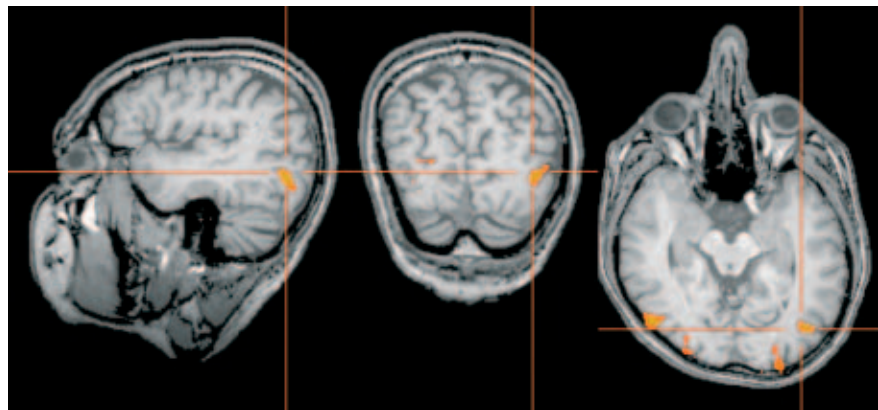
Abb. 5: Koregistrierung der zweidimensional gemessenen Aktivierungen (hier: das extrastriäre bewegungssensitive visuelle Areal V5) mit einer dreidimensionalen MRT-Aufnahme der Anatomie.
