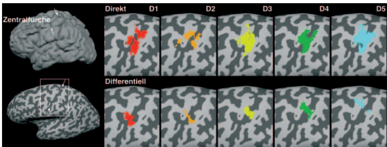
Abb. 12: Fingerrepräsentationen im primären motorischen Handareal (M1) nach Segmentierung und Entfaltung des Gehirns (vgl. Abb. 6). (Oben) Während eine Bewegung gegen Ruhe zu starken Überlappungen führt, ergibt (unten) ein differentieller Vergleich unterschiedlicher Fingerbewegungen eine geordnete somatotopie Reihung von D1: Daumen, D2: Zeigefinger, D3: Mittelfinger, D4: Ringfinger und D5: kleiner Finger. Verändert aus Dechent und Frahm (2003).
