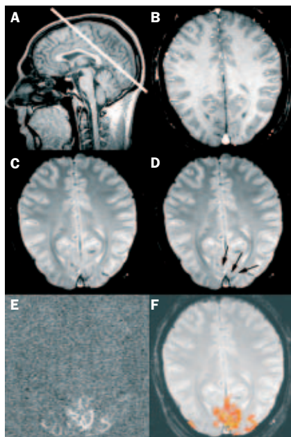
Abb. 2: Die Elemente eines fMRT-Experimentes (hier: visuelle Stimulation mit einem Schachbrettmuster im Vergleich zu einem grauen Bild) betreffen: (A) die Wahl eines Volumens (hier: eine Schicht durch den okzipitalen Kortex), (B) die MRT-Darstellung der Anatomie, (C) die Aufnahme einer dynamischen Zeitserie von MRT-Bildern während der Kontrollbedingung und (D) während der Stimulationsbedingung (Pfeile: Bereiche mit erhöhter Signalintensität im okzipitalen Kortex), (E) eine Grauwert-Karte der berechneten Korrelationskoeffizienten (hell: hoch korreliert, grau: nicht korreliert, dunkel: entgegengesetzt korreliert) und (F) die Überlagerung einer farbkodierten Karte der statistisch signifikanten Aktivierungen mit einem geeigneten Referenzbild.
