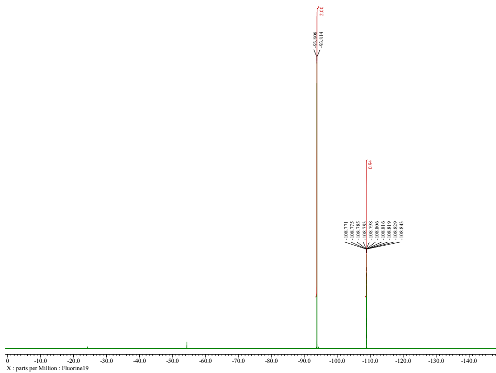
2,2-Difluoro-2-(4-fluorophenyl)ethan-1-ol (5c)
