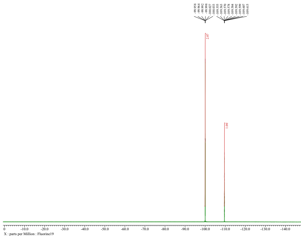
2,2-Difluoro-2-(4-fluorophenyl)ethan-1-amine (1c)
