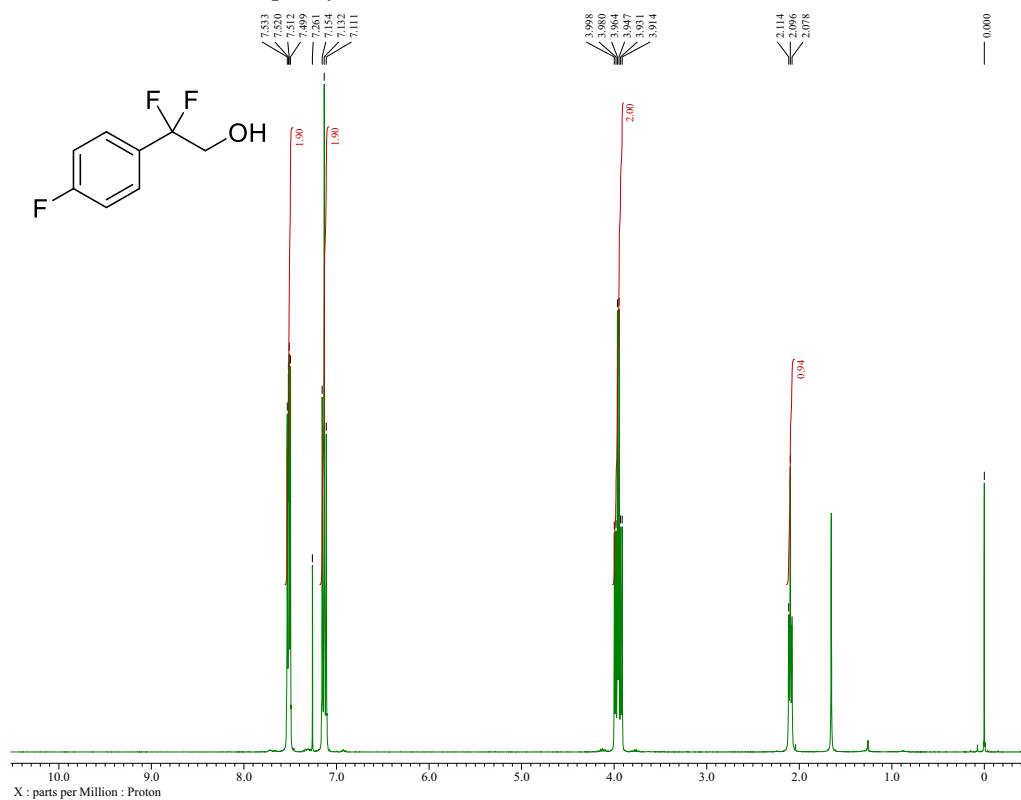
2,2-Difluoro-2-(4-fluorophenyl)ethan-1-ol (5c)
