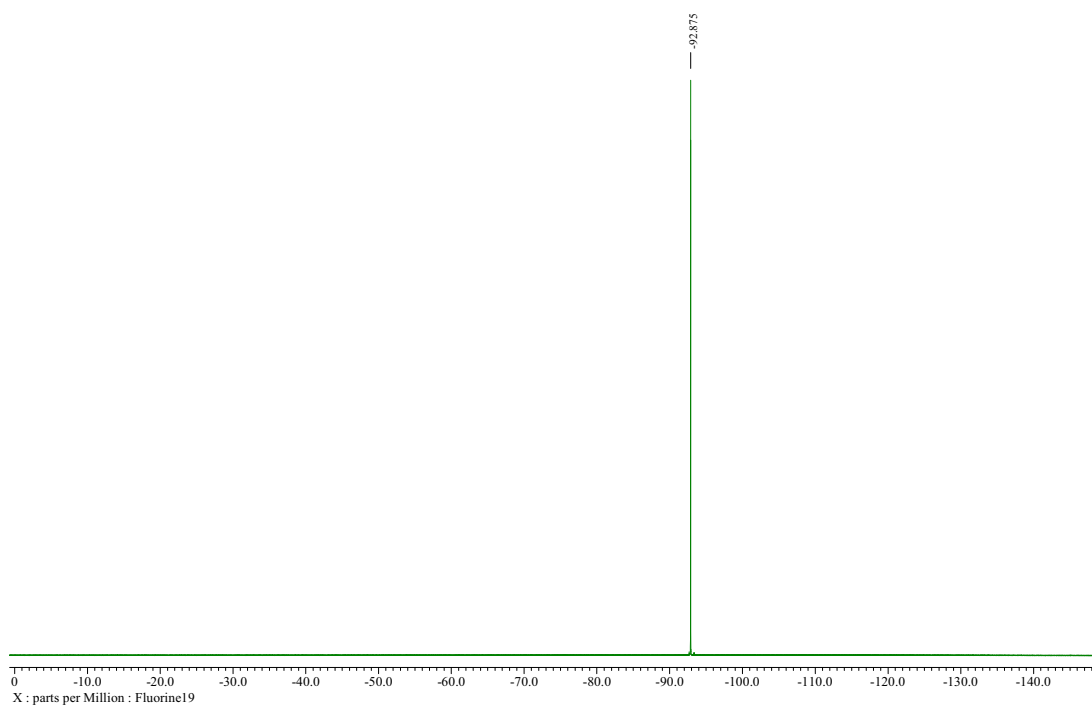
2-(4-(Benzyloxy)phenyl)-2,2-difluoroethan-1-ol (5b)
