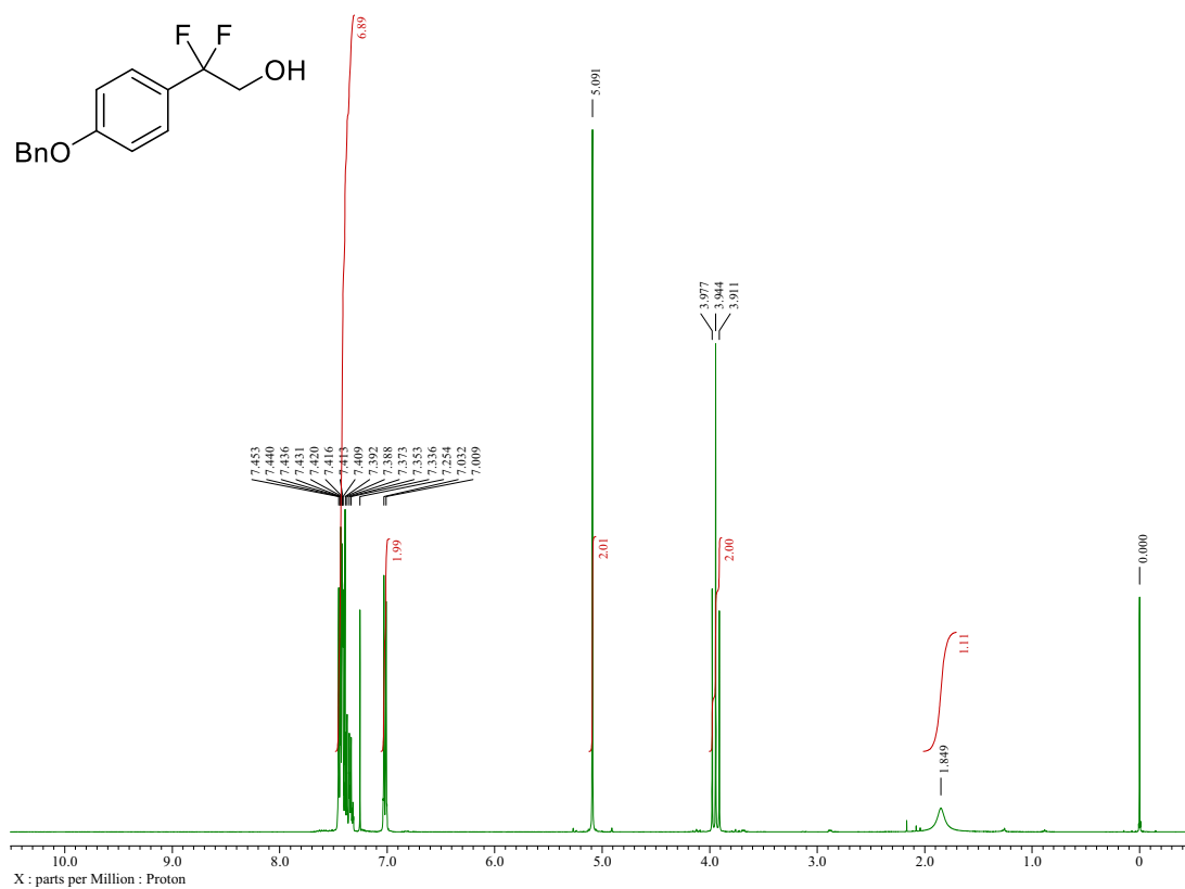
2-(4-(Benzyloxy)phenyl)-2,2-difluoroethan-1-ol (5b)
