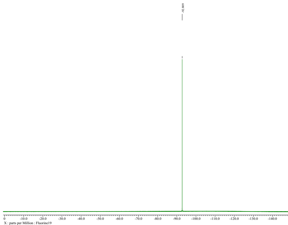
2,2-Difluoro-2-(4-methoxyphenyl)ethan-1-ol (5a)
