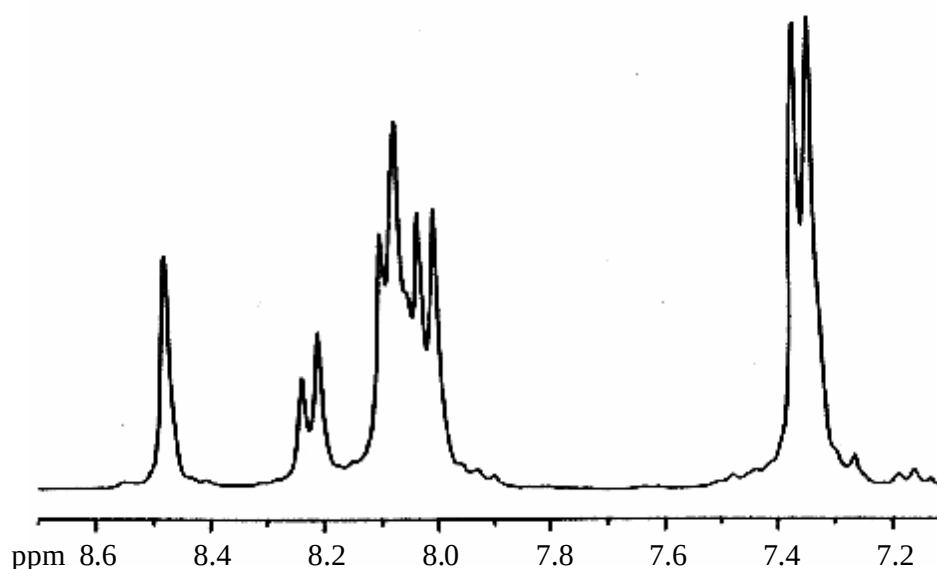
Fig. 3. ^1\text{H} NMR spectrum of 2,6-PEKEKNK.
