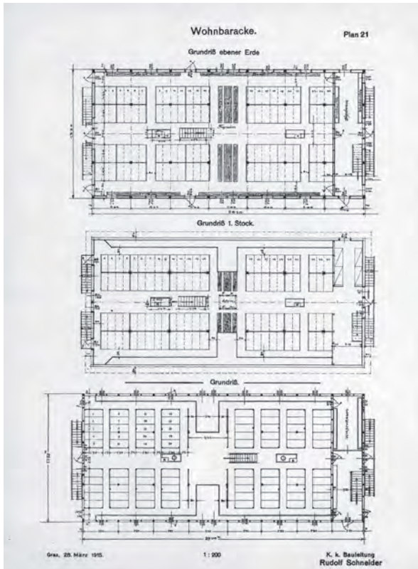
64 Flüchtlingslager Wagna, Steiermark, Österreich, Wohnbaracke für ca. 500 Personen (aus: Franz Haimel, Flüchtlingslager Wagna, Graz 1915).
