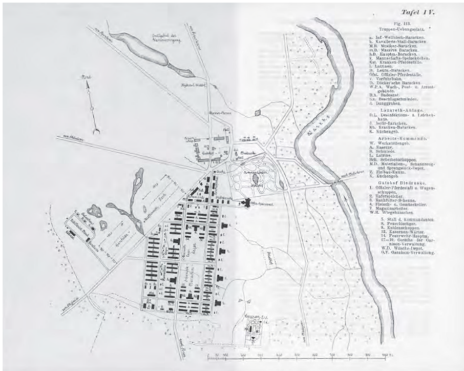
11 Plan eines Barackenlagers für Truppenübungen (aus: Baukunde des Architekten , Berlin 1900, 2. Bd., 4. T., 2. Aufl.).
