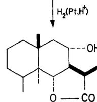
Deoxotetrahydroartemisin
